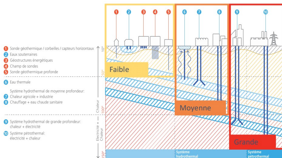
Types de géothermie (source : OFEN)
